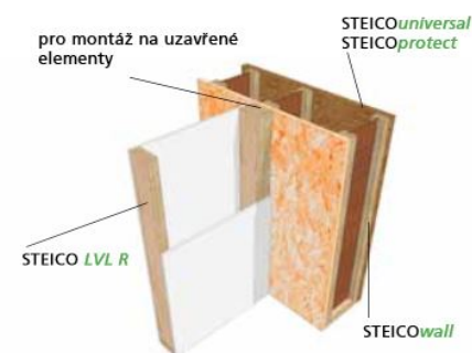
W3 Připojení vnitřní stěny na obvodovou
