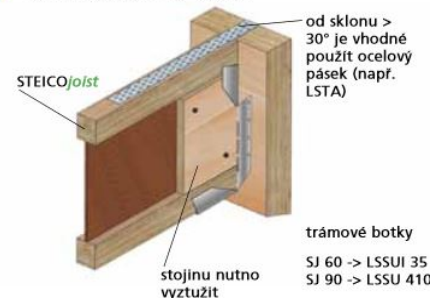
D2 Boční upevnění na vaznici
