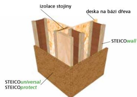
W1 vnější roh
