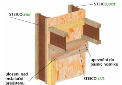
F2 Připojení stropu v provedení baloon-framing
