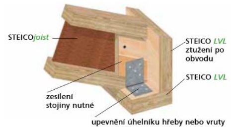
D6 Vodorovné uložení
